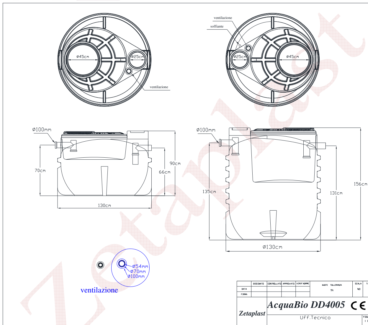
Fig.6 – Schema tecnico
