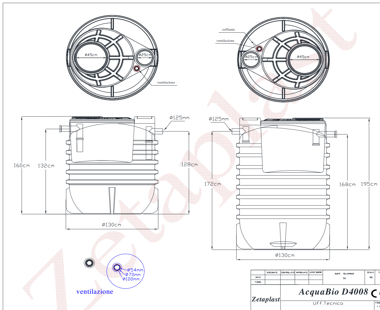
Fig.6 – Schema tecnico
