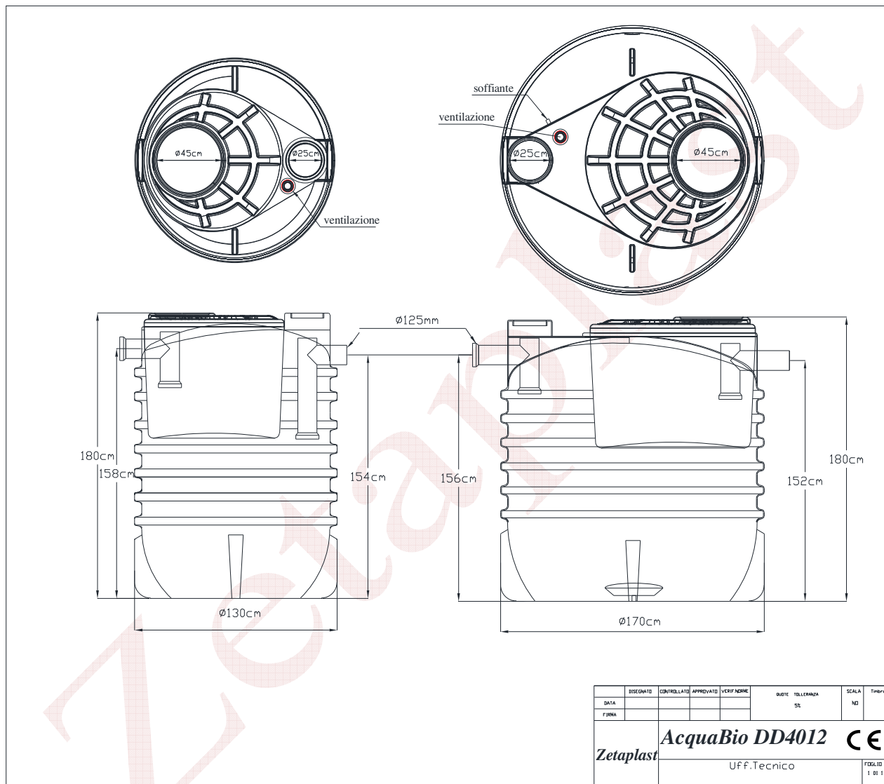
Fig.6 – Schema tecnico
