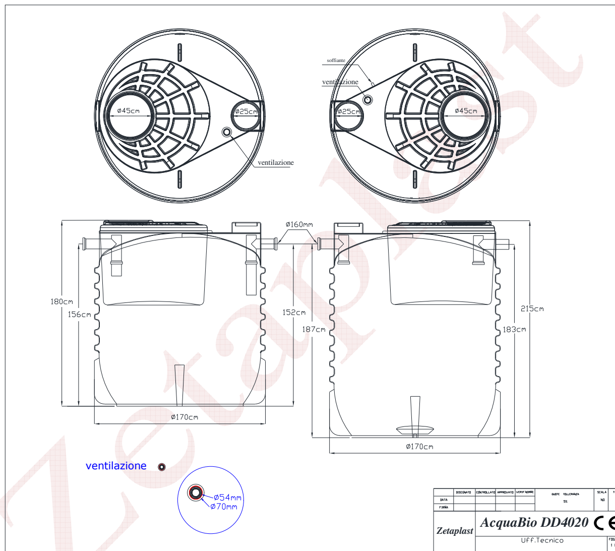
Fig.6 – Schema tecnico
