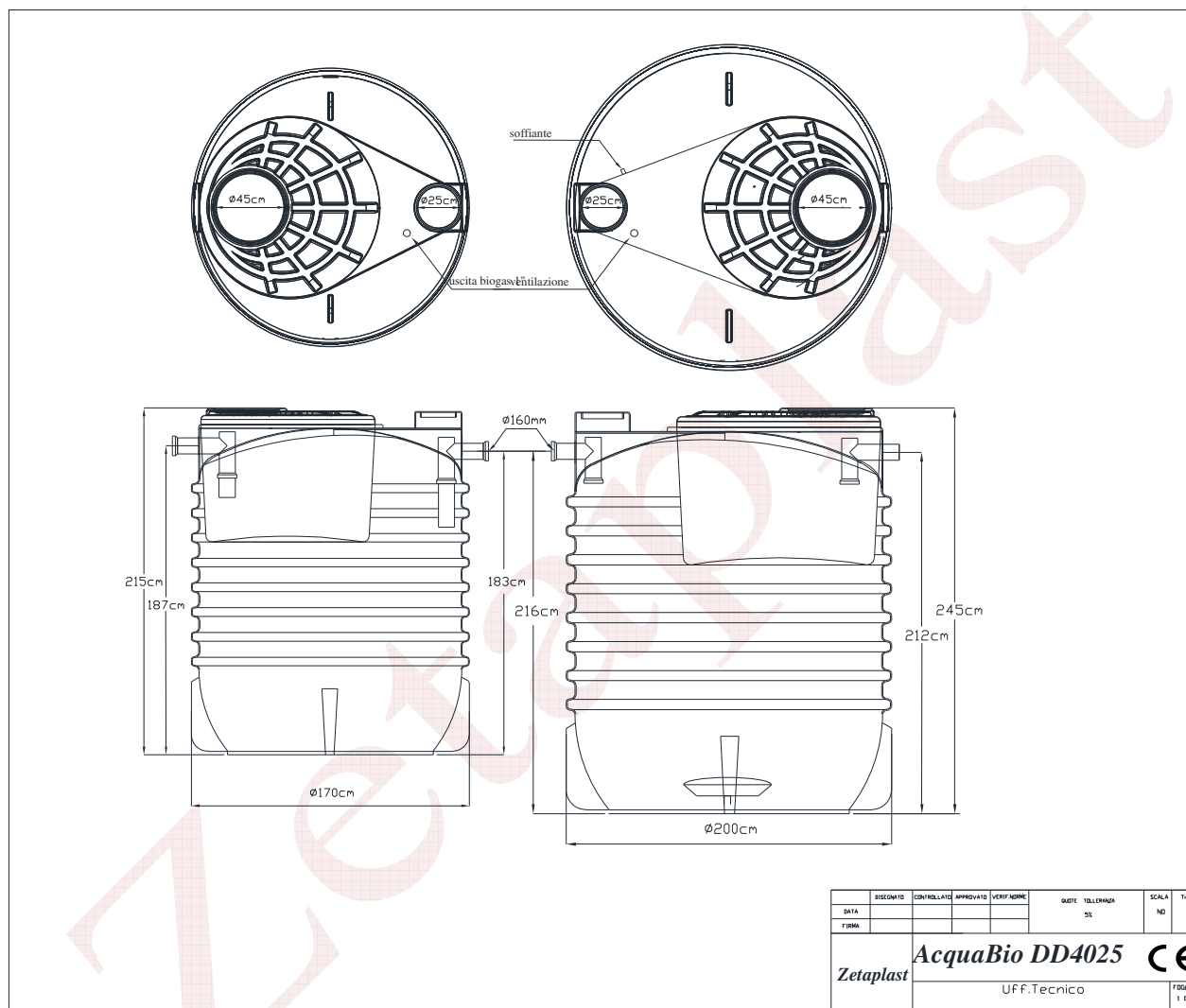
Fig.6 – Schema tecnico
