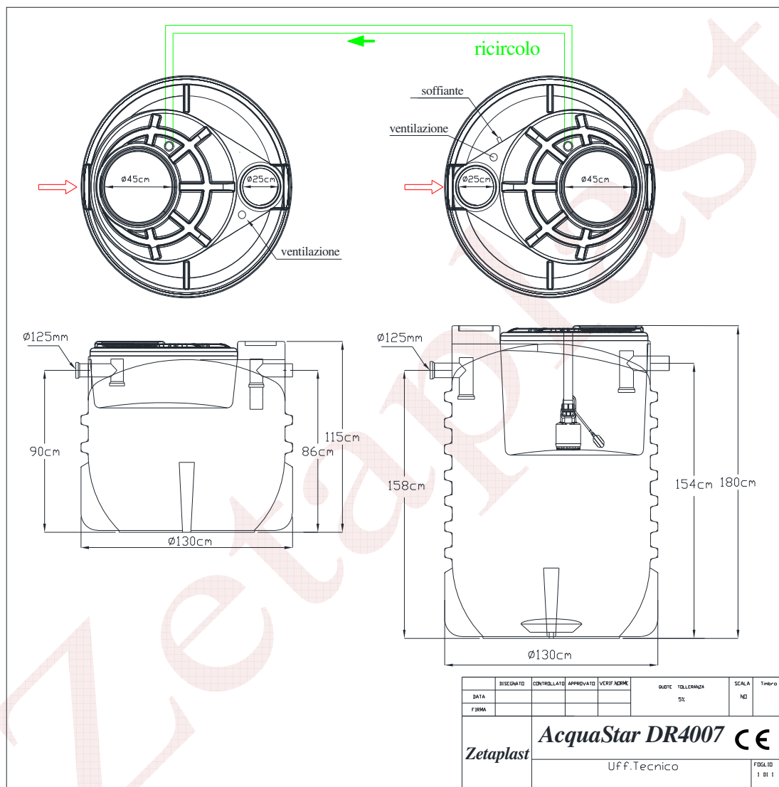
Fig.6 – Schema tecnico
