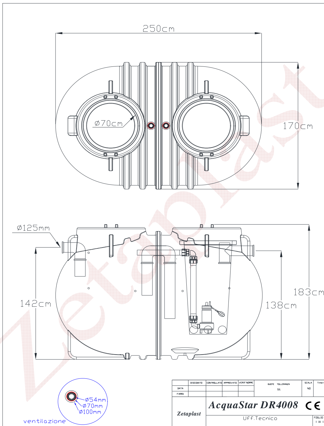
Fig.6 – Schema tecnico
