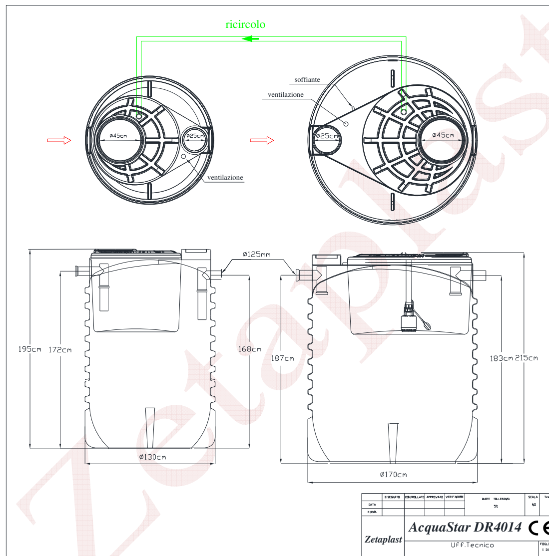
Fig.6 – Schema tecnico
