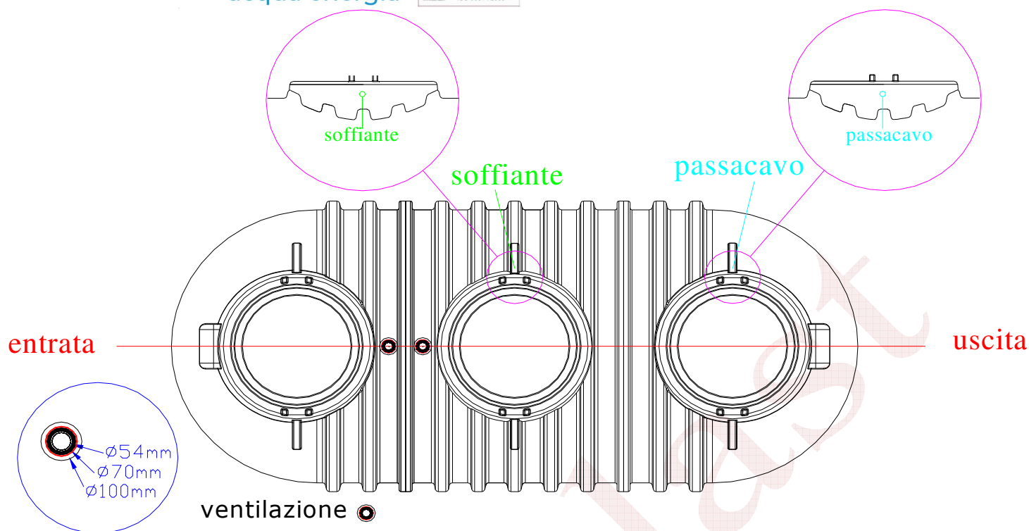
Fig.2 – Posizionamento collegamenti biogas-ventilazione, soffiante e ricircolo
