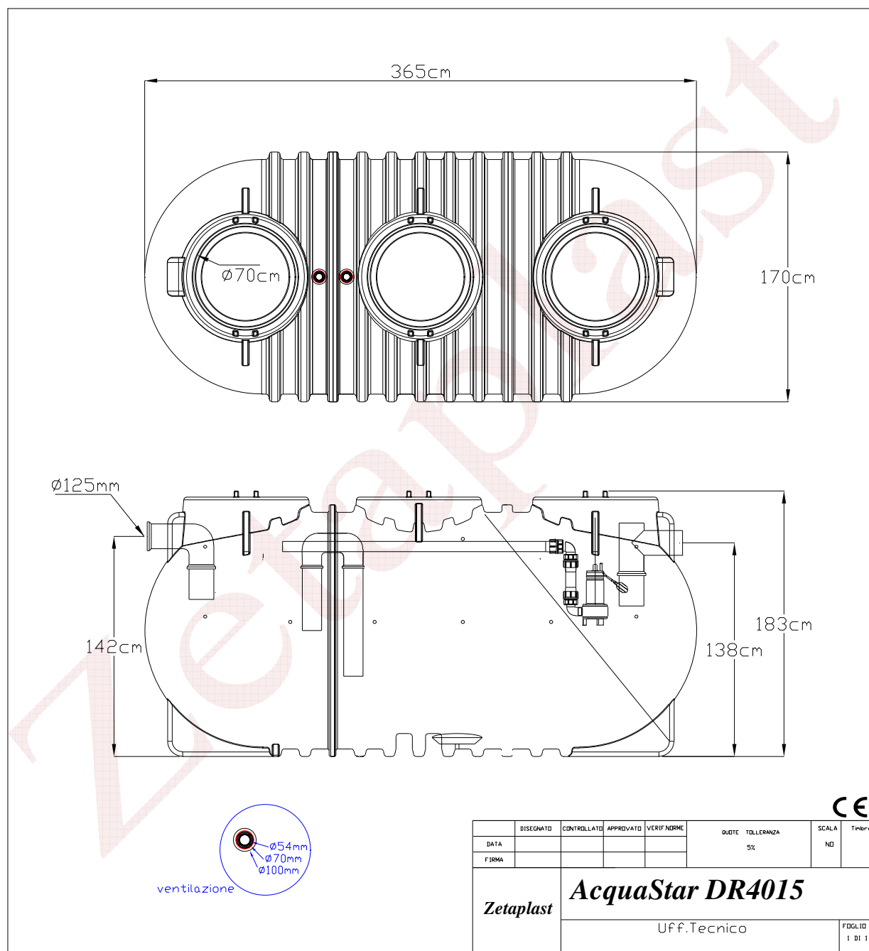
Fig.6 – Schema tecnico
