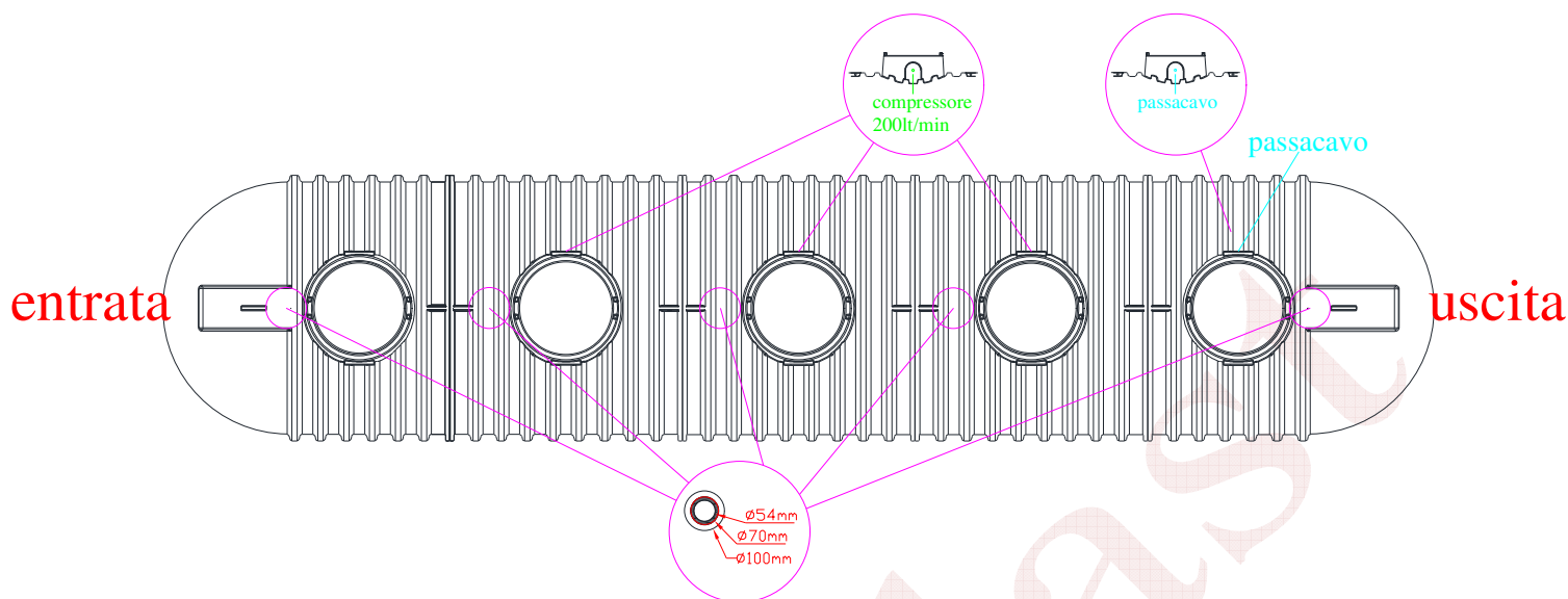
Fig.2 – Posizionamento collegamenti biogas-ventilazione, soffiante e ricircolo
