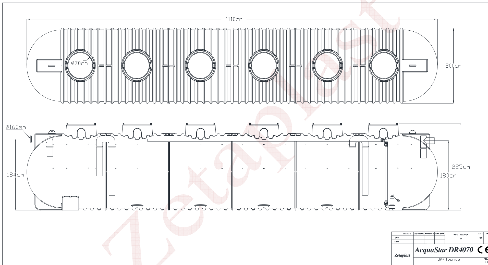
Fig.6 – Schema tecnico
