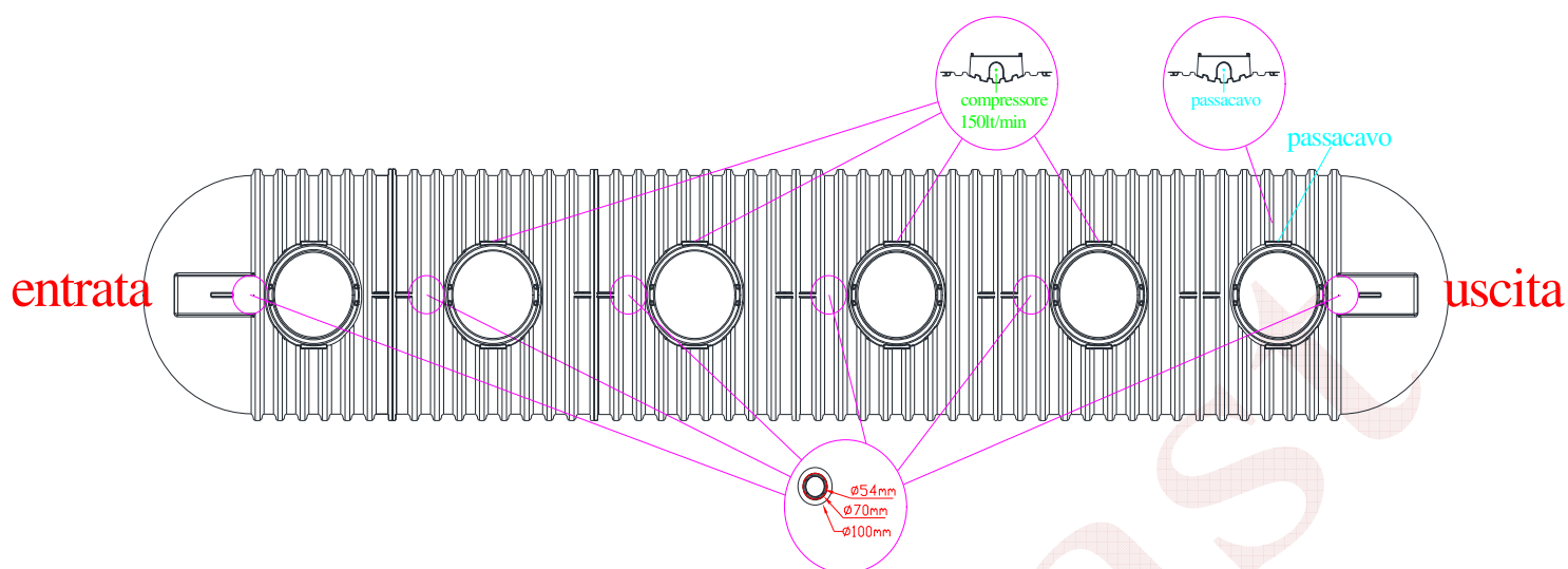
Fig.2 – Posizionamento collegamenti biogas-ventilazione, soffiante e ricircolo
