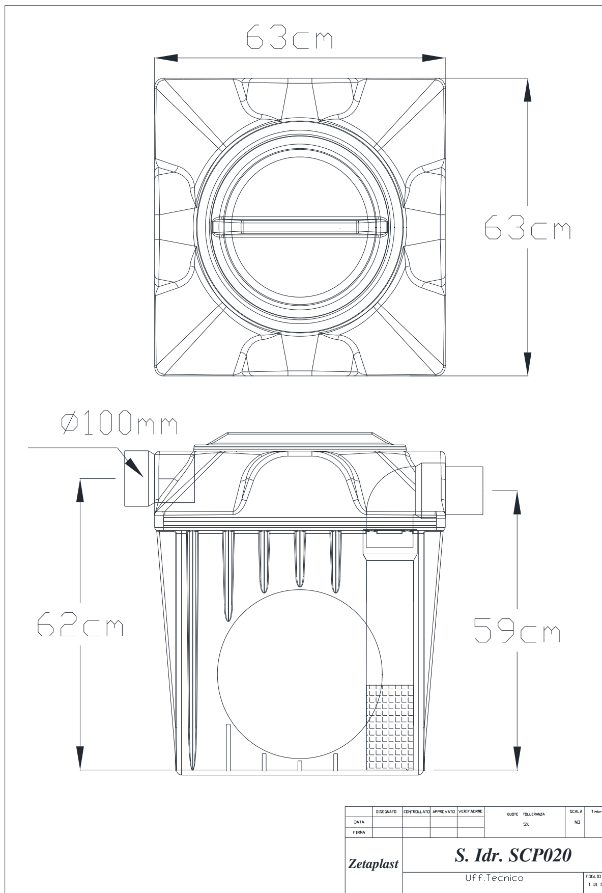
Fig.2 – Schema tecnico
