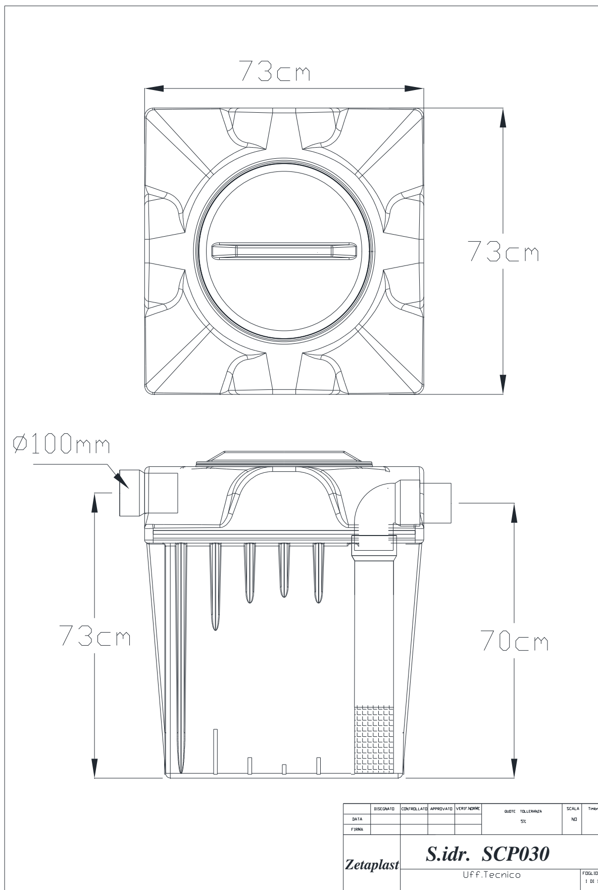
Fig.2 – Schema tecnico
