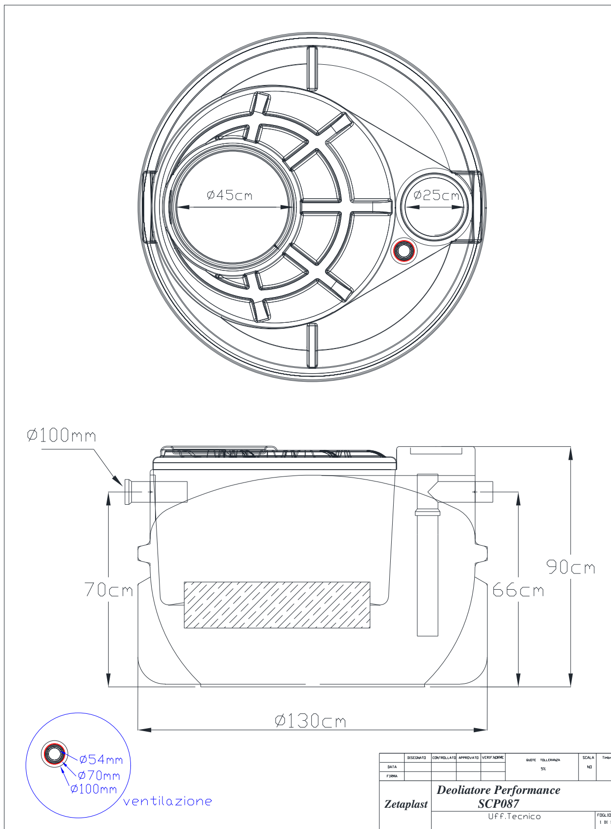
Fig.2 – Schema tecnico
