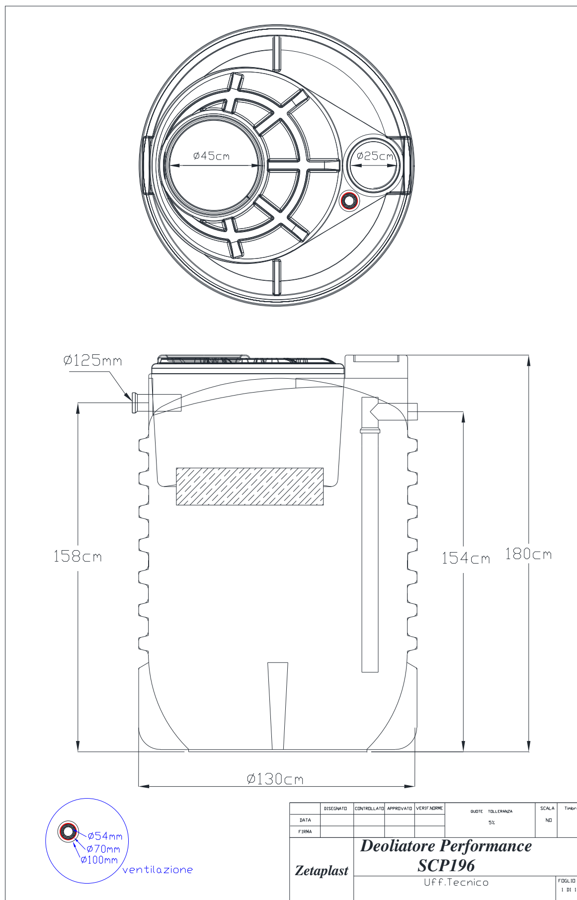
Fig.2 – Schema tecnico
