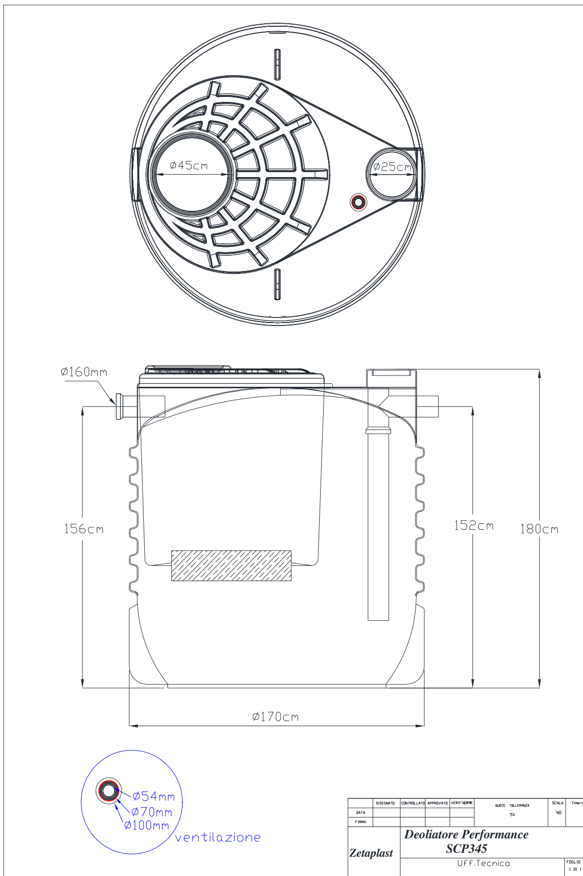
Fig.2 – Schema tecnico
