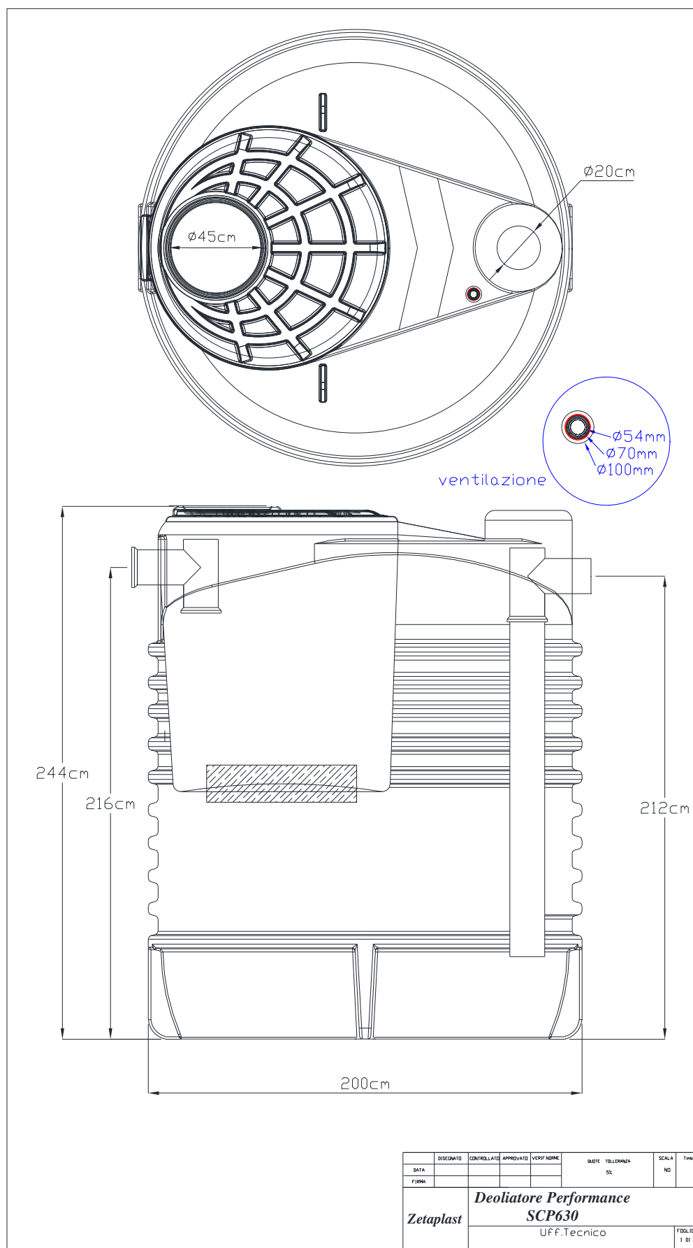
Fig.2 – Schema tecnico
