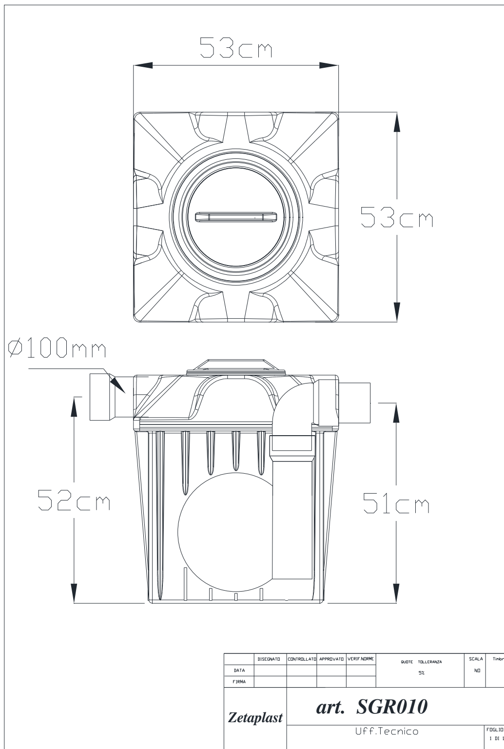
Fig.2 – Schema tecnico
