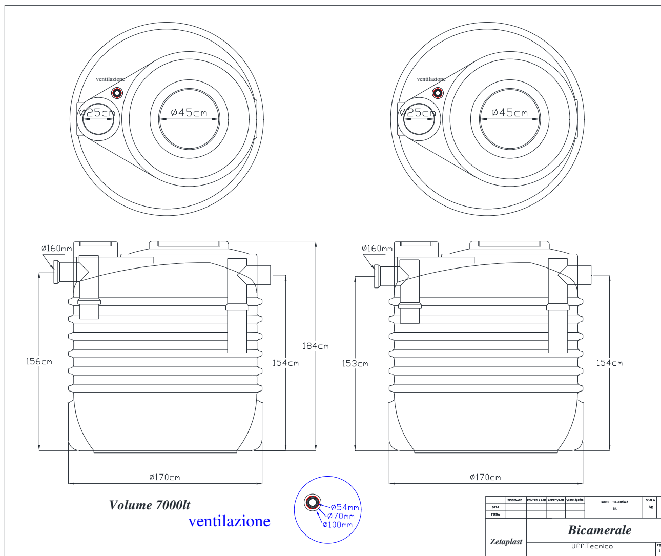
Fig. 8 - Bicamerale
